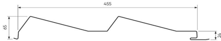
Solape lateral (sistema de fijación oculta) Side lap (hidden fixing system) Recouvrement latéral (système de fixation cachée)
