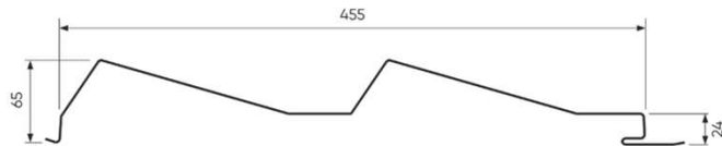
Solape lateral (sistema de fijación oculta) Side lap (hidden fixing system) Recouvrement latéral (système de fixation cachée)
